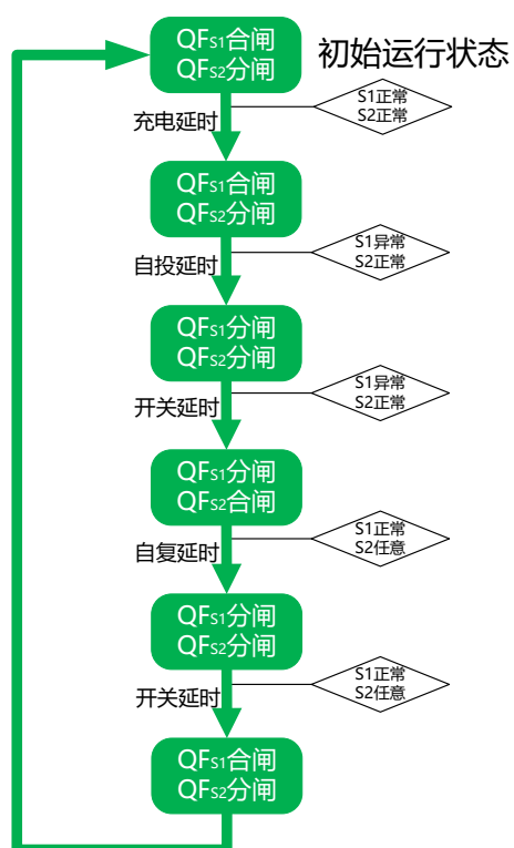
图三 2B 型控制器自投自复流程
