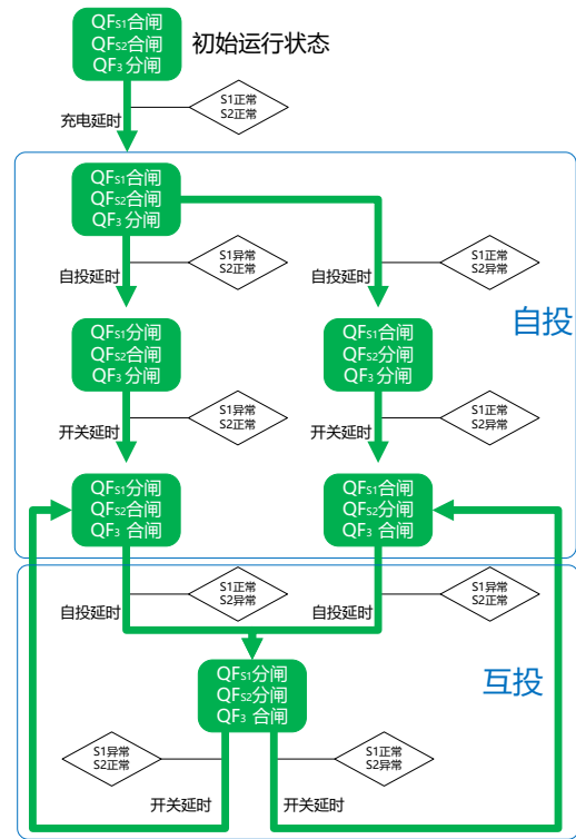
图九 3B 型控制器自投不自复（互投）流程
